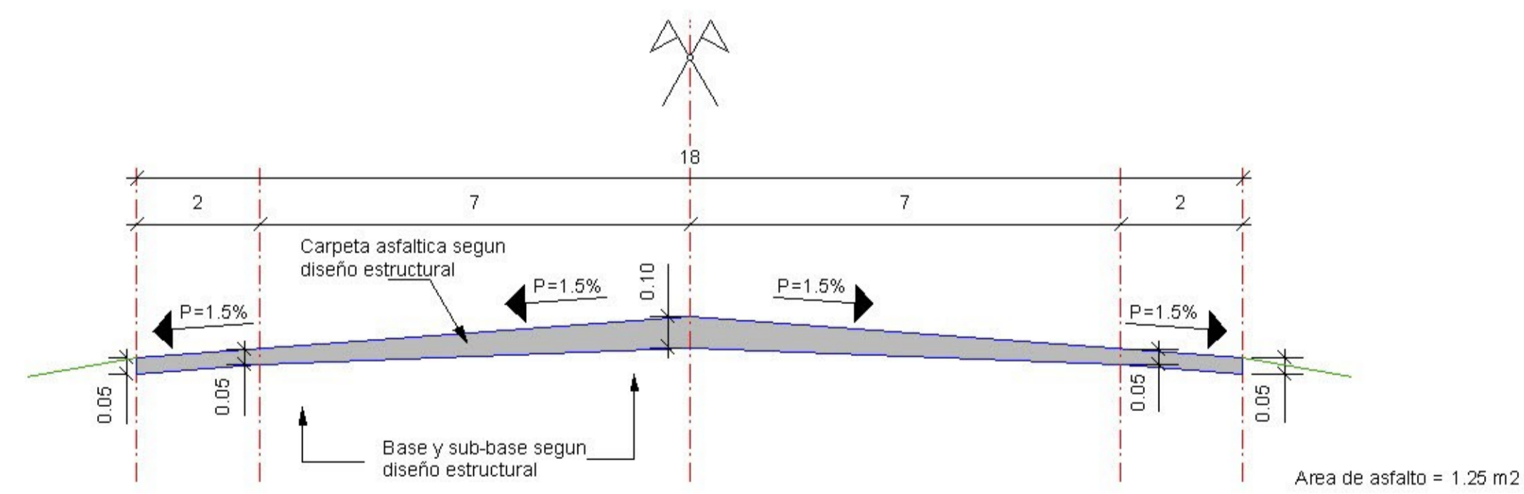
2 GABARITO TIPICO DE PISTA
